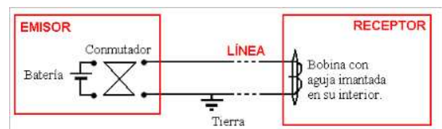
Figura 4. Esquema Eléctrico del Telégrafo de Gauss.
