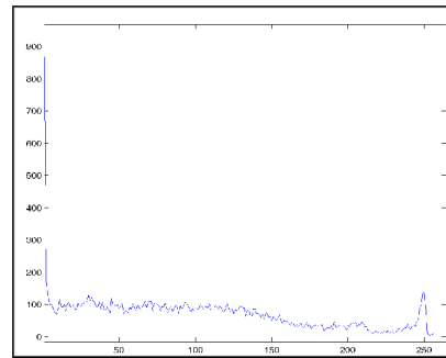
Histograma de grises del iris recortado: aquí deberíamos encontrar los umbrales para localizar el iris. Funciona casi cualquier par que empiece después del pico en cero (pupila negra) y acabe antes del pico en trono al 255 (restos de esclerótica).
